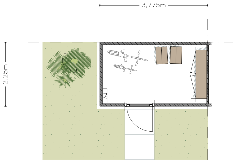
BEGANE GROND
